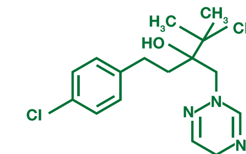
Tebuconazol
